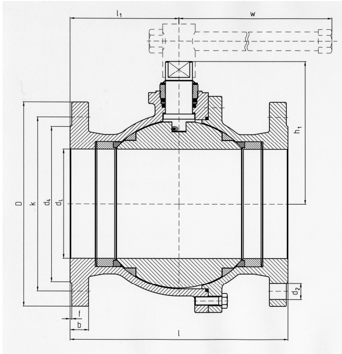
Bild 2: Kugelhahn mit vollem Durchgang und Flanschanschluß nach DIN EN 1092-1, Form B1 (DIN 2526 Form C); Baulänge: Grundreihe 27 nach EN 558-1 (F18 nach DIN 3202 Teil 1)
