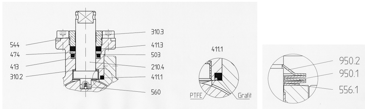
Variante 3: Keilring-Abdichtung
