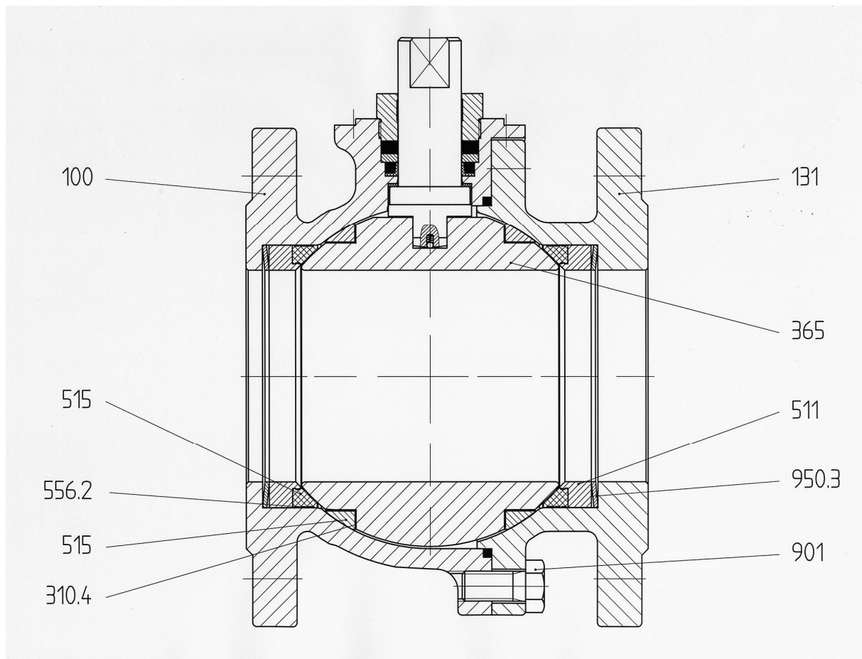
Bild 1: Kugelhahn mit vollem Durchgang
